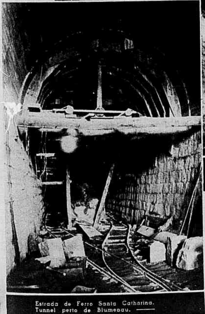
Estrada de Ferro Santa Catharina. (Construção de ponte sobre o rio Itajahy Assú (1930) e de acessos e tunnel 1930).
