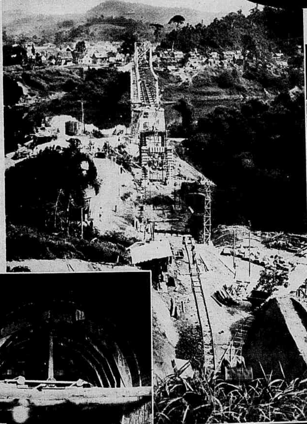
Estrada de Ferro Santa Catharina. (Construção de ponte sobre o rio Itajahy Assú (1930) e de acessos e tunnel 1930).
